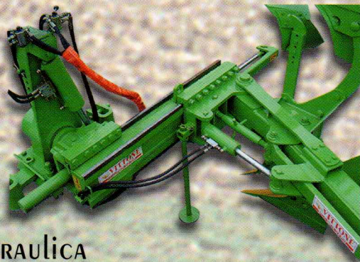
PENTAVOMERE ENTRO-FUORISOLCO PIEGABILE
